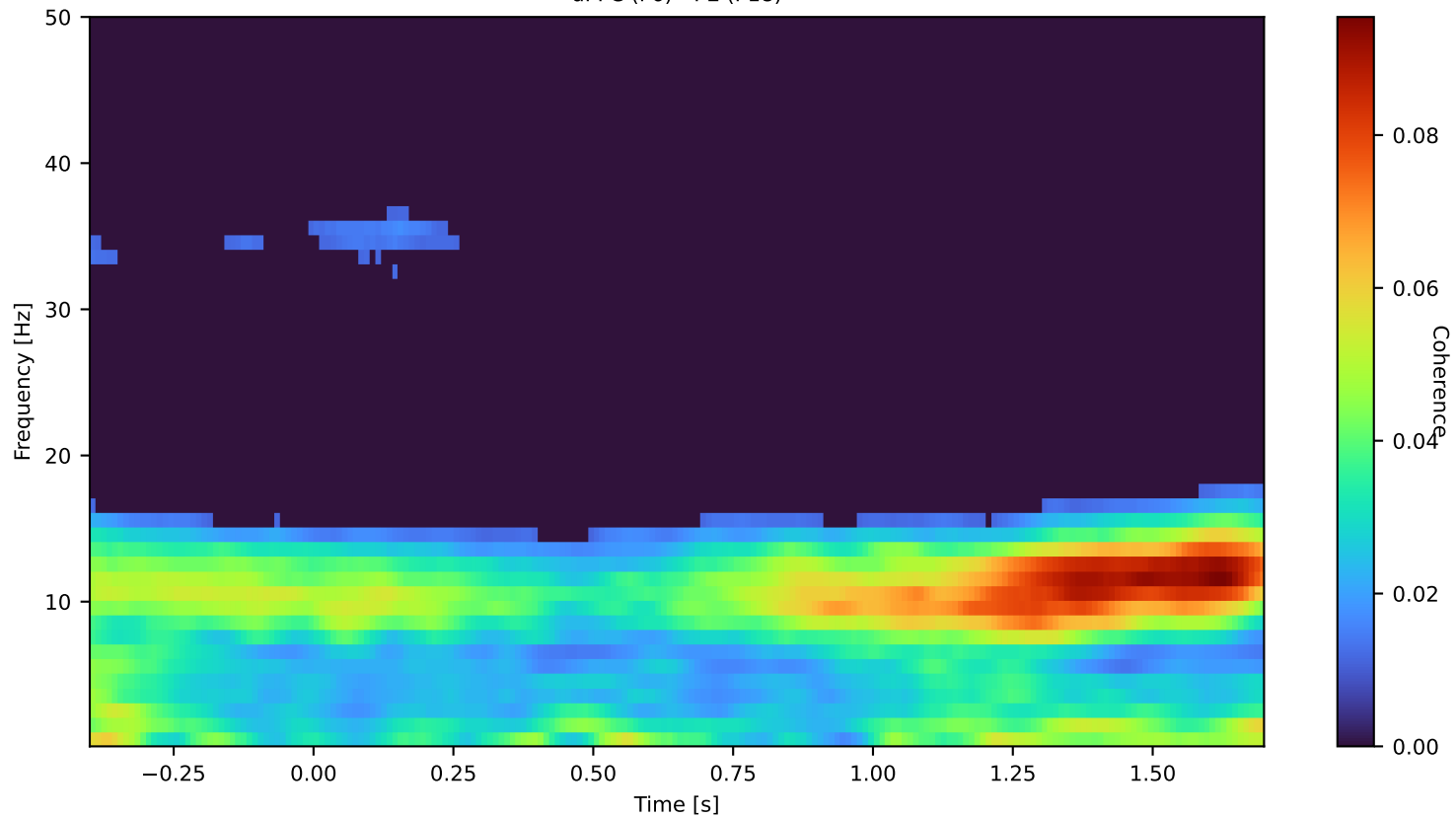
dPFC (F6) - PE (P18)
